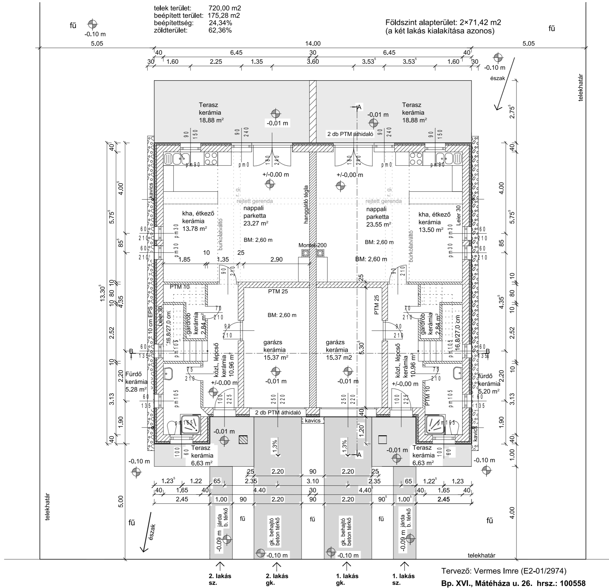
E - 3 Földszint alaprajz M 1 : 100 (A3) 2015.05.05.
