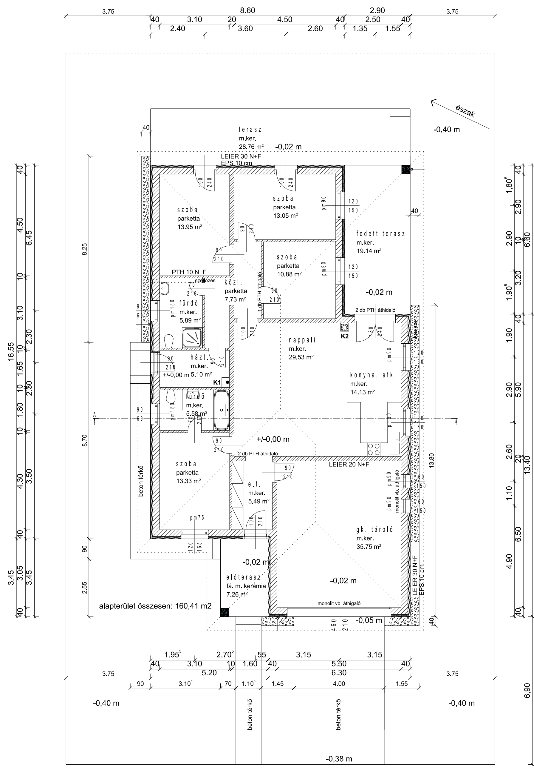
E - 3 Földszint alaprajz M 1 : 100 2014.04.29.
