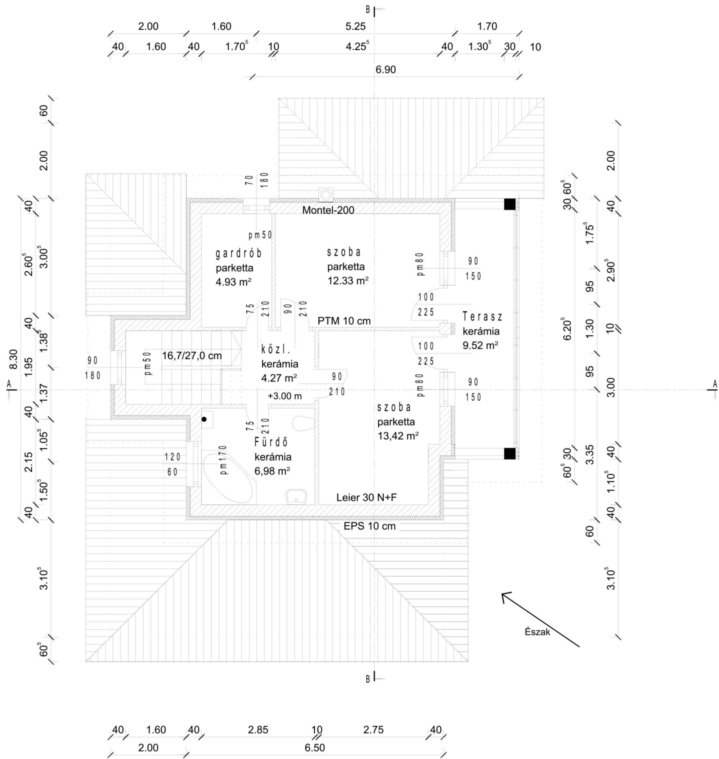
E - 3 Emelet alaprajz M 1:100 (A3) 2015.06.21.
