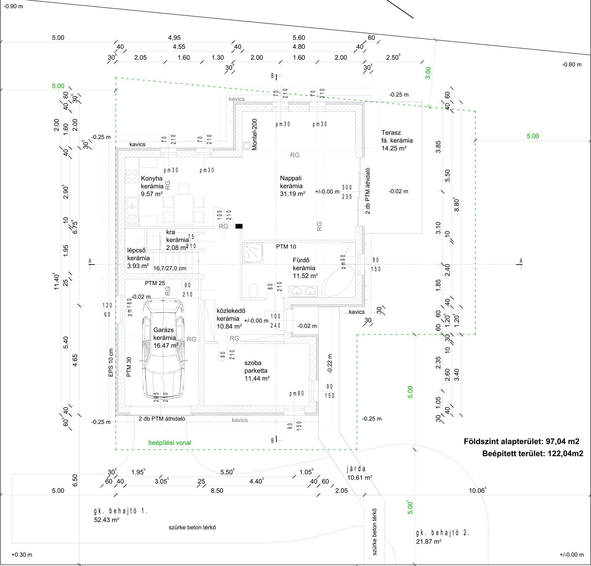
E - 2 Földszint alaprajz (A3) M 1:100 2015.06.21.
