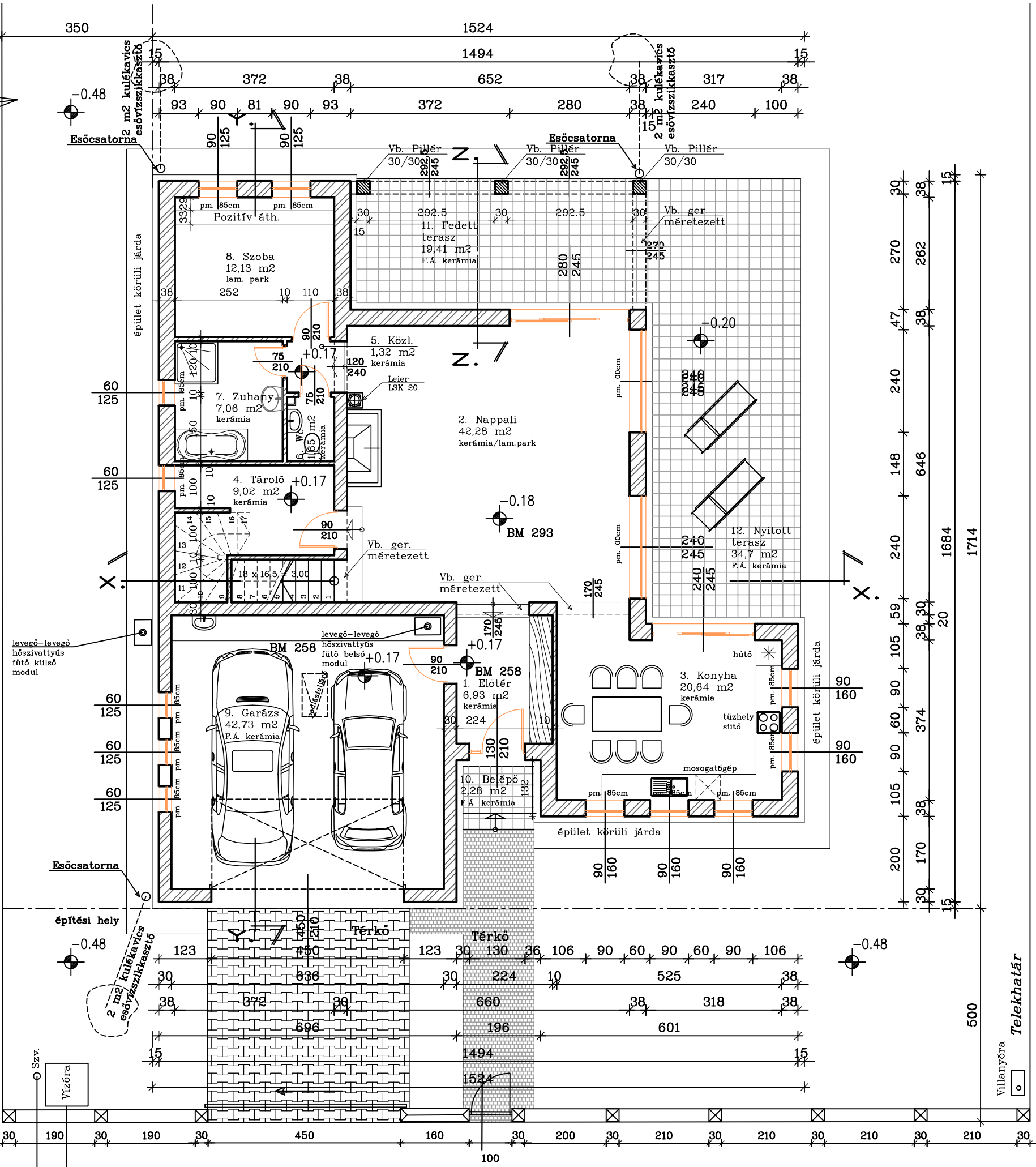
FÖLDSZINTI ALAPRAJZ M 1 : 100
